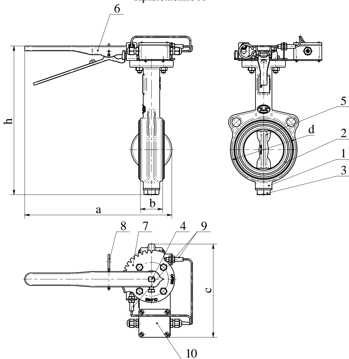
Рисунок А.1 - Затвор дисковый DN 50 (65, 80, 100, 125, 150, 200)
