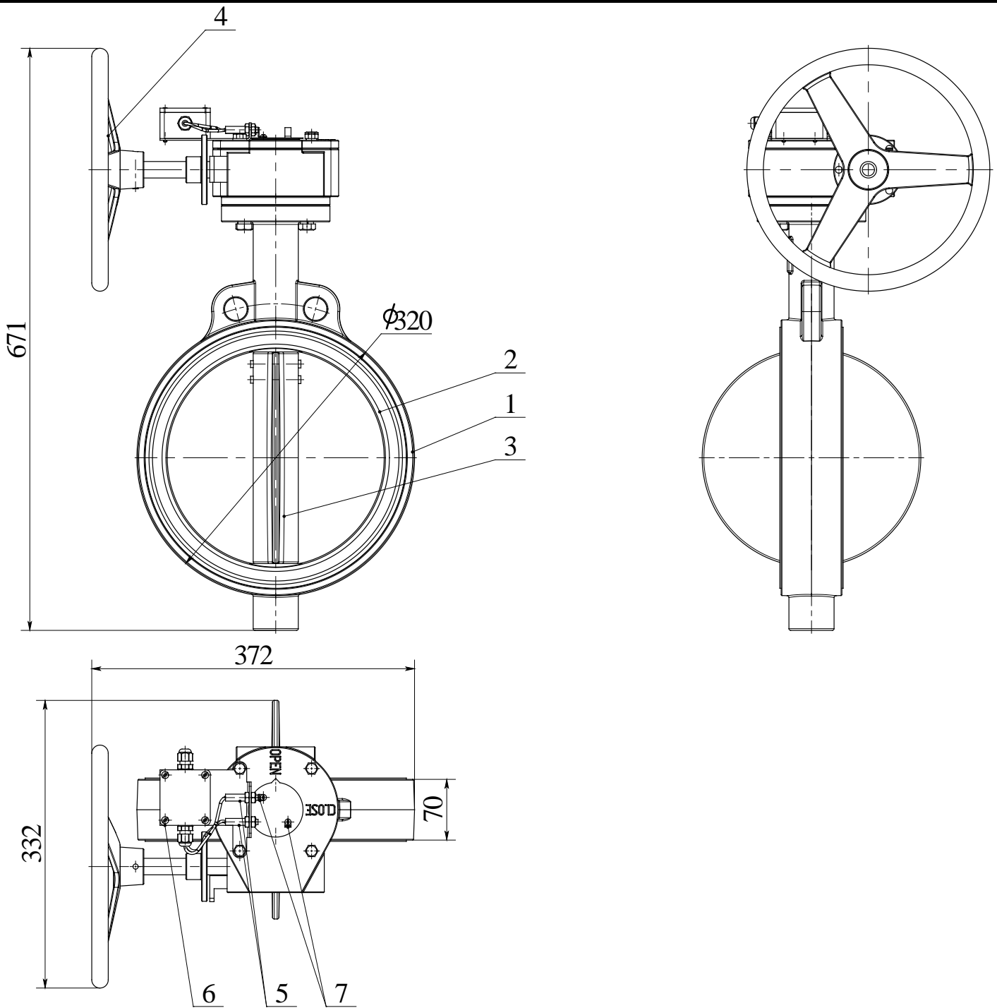
Рисунок А.2 - Затвор дисковый DN 250
