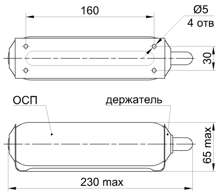
Рисунок 2.1 - ОСП с держателем защелка
