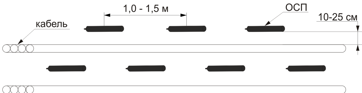
Рисунок 3 - Варианты размещения ОСП
